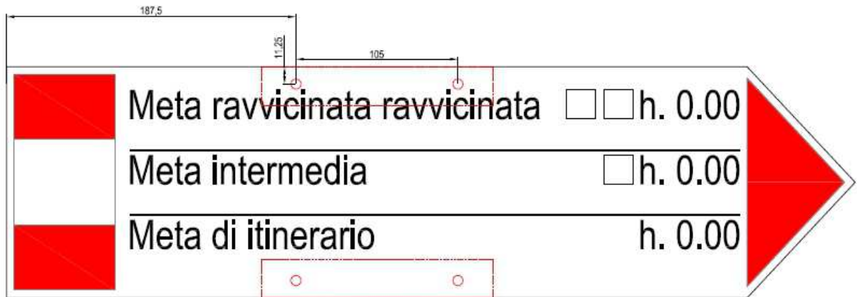
Figura 3: Schema di posizionamento dei buchi di fissaggio sulla tabella per il collare a ponte.
